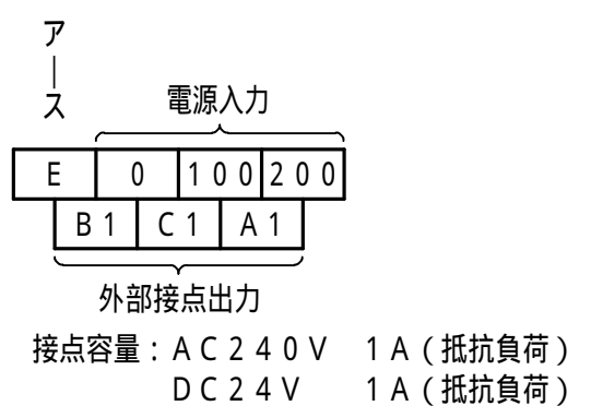
端子台詳細図
